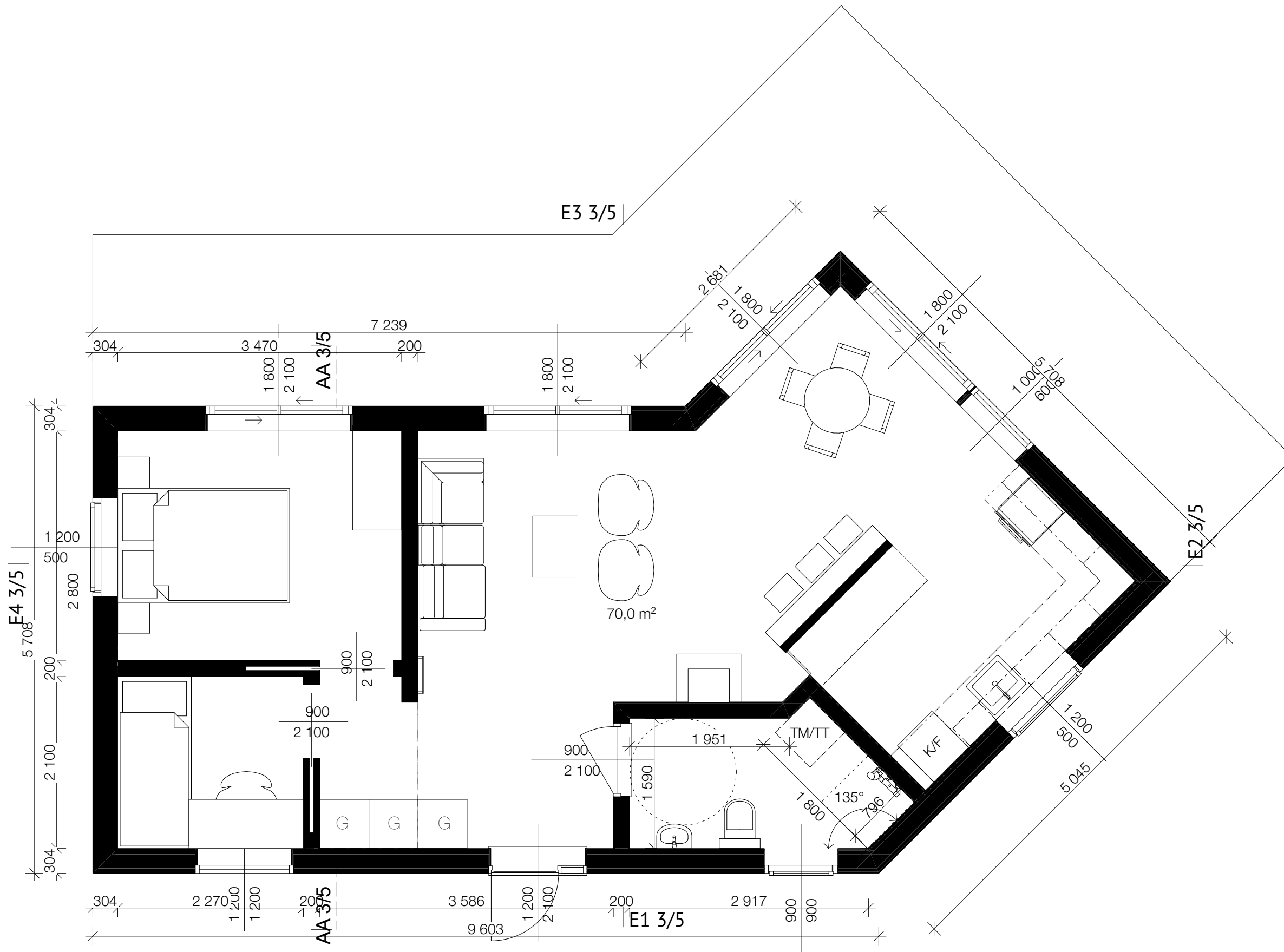
HUS 3/5 ENTRÉVÅNING 1:50
